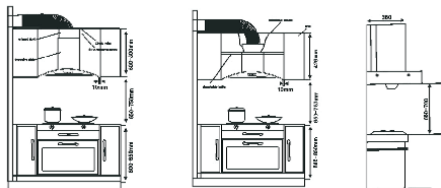
Dimensi dan letak plate untuk instalasi overhead
